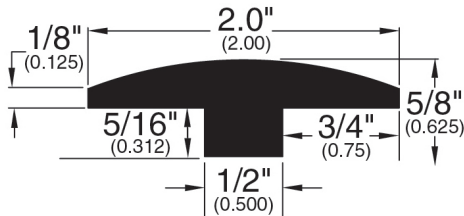
T-Mold (002)
