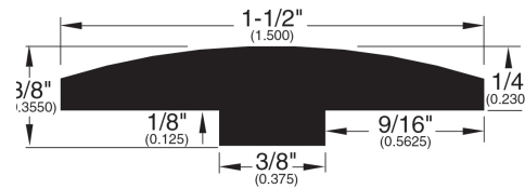
T-Mold (702)
